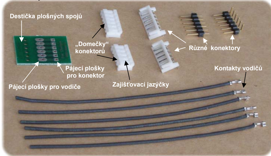
Příklady osazení konektoru pro servokabel vašich článků
